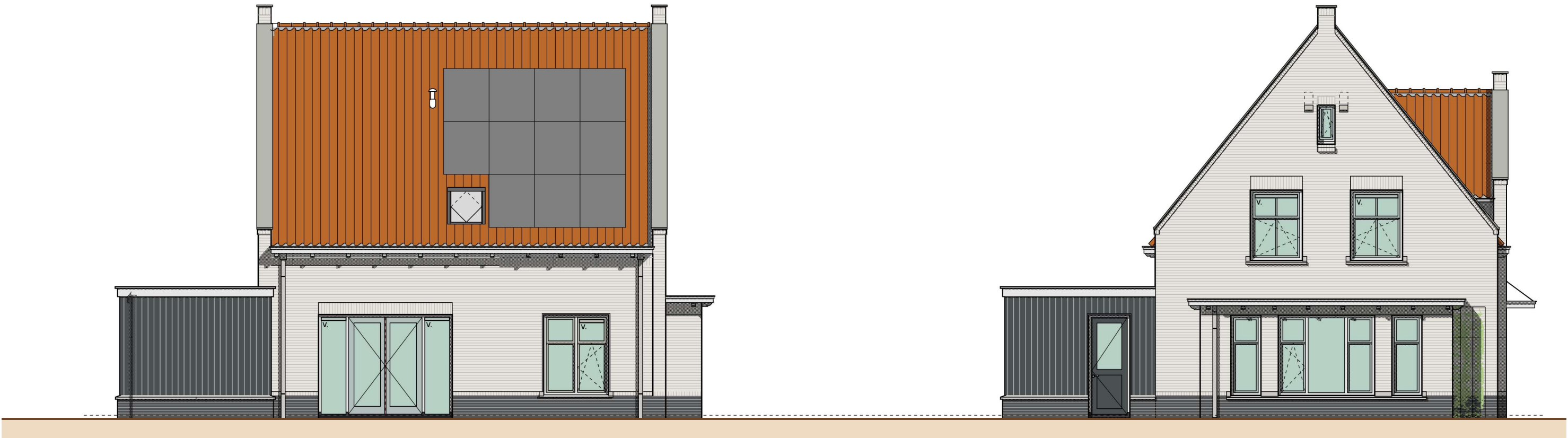
Achtergevel
